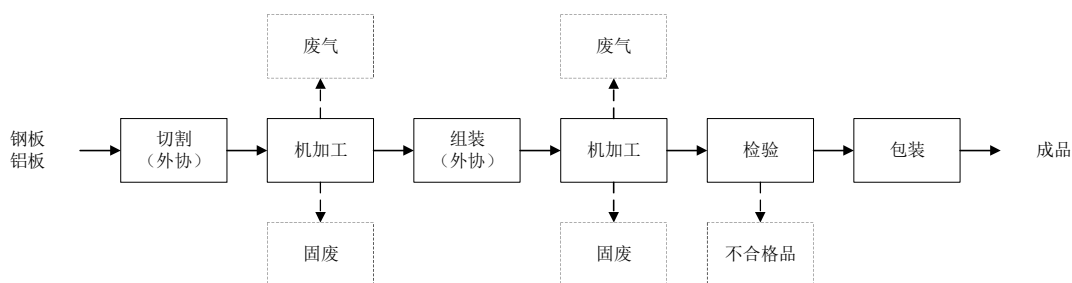
图 5-1 本项目生产工艺及排污点示意图
