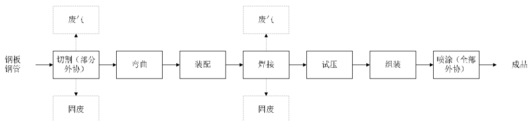
图 5-1 本项目生产工艺及排污点示意图
